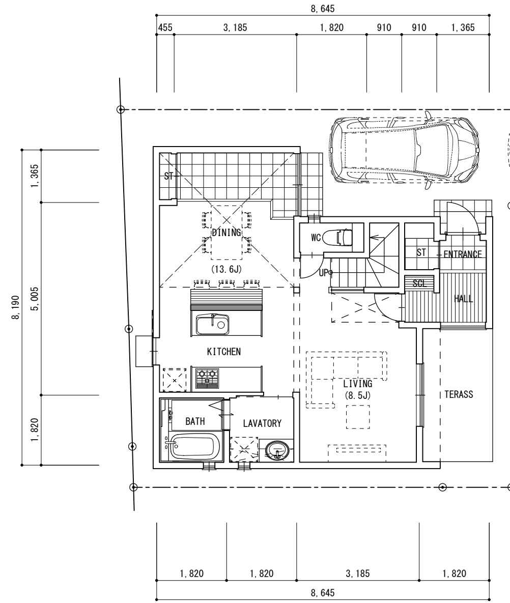
1階平面図
