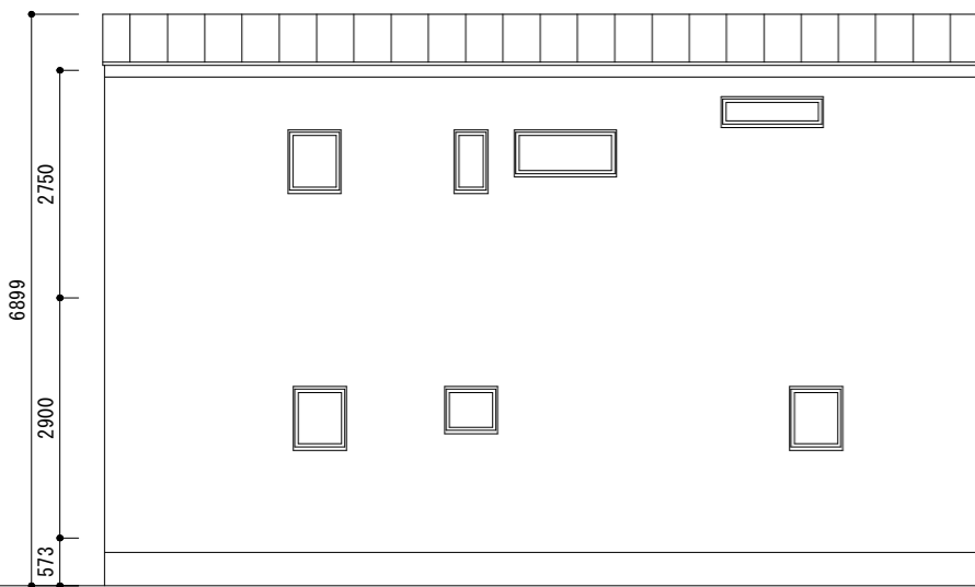
北 立面
