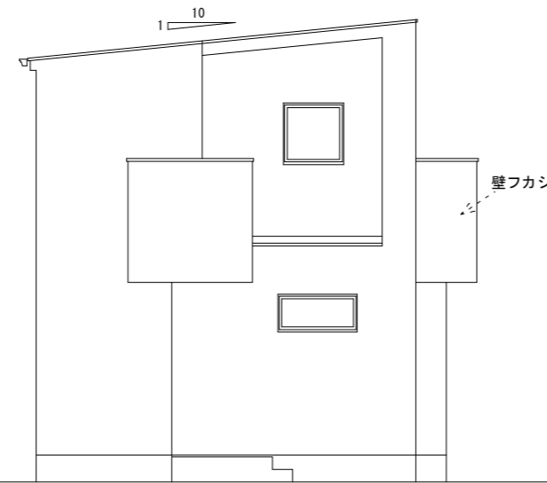
西 立面
