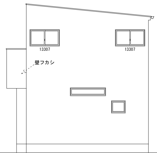
東 立面
