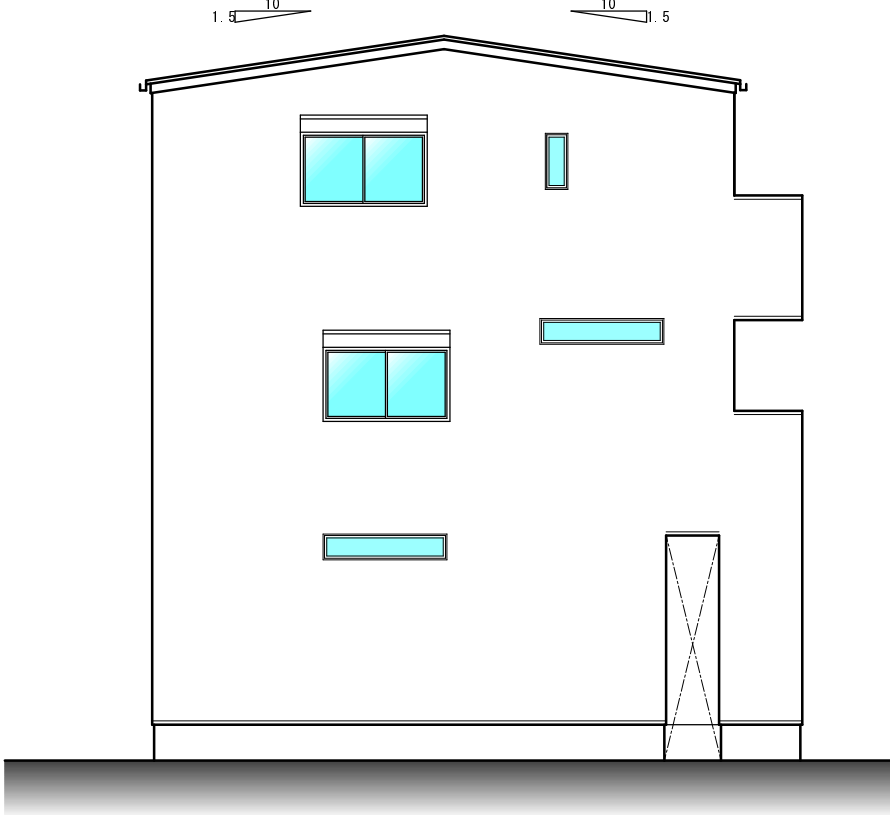
南側立面図 1/100
