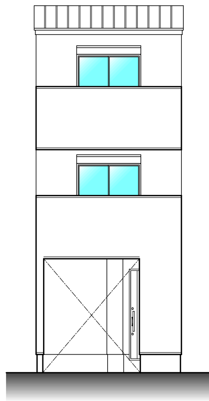
東側立面図 1/100
