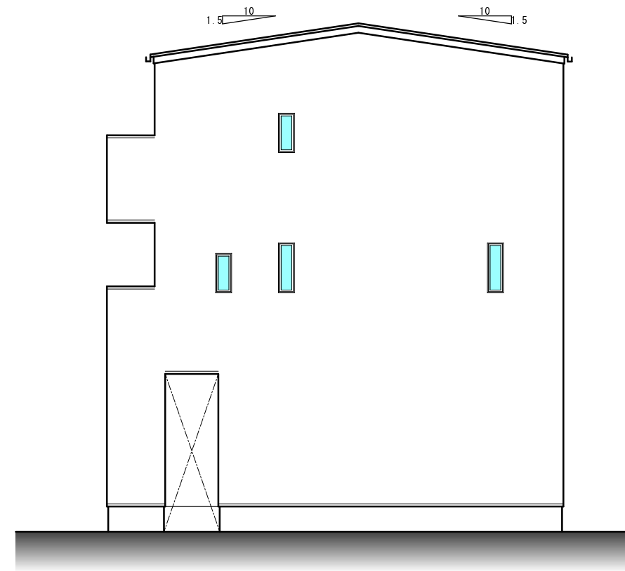
北側立面図 1/100
