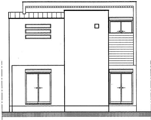
南立面图
