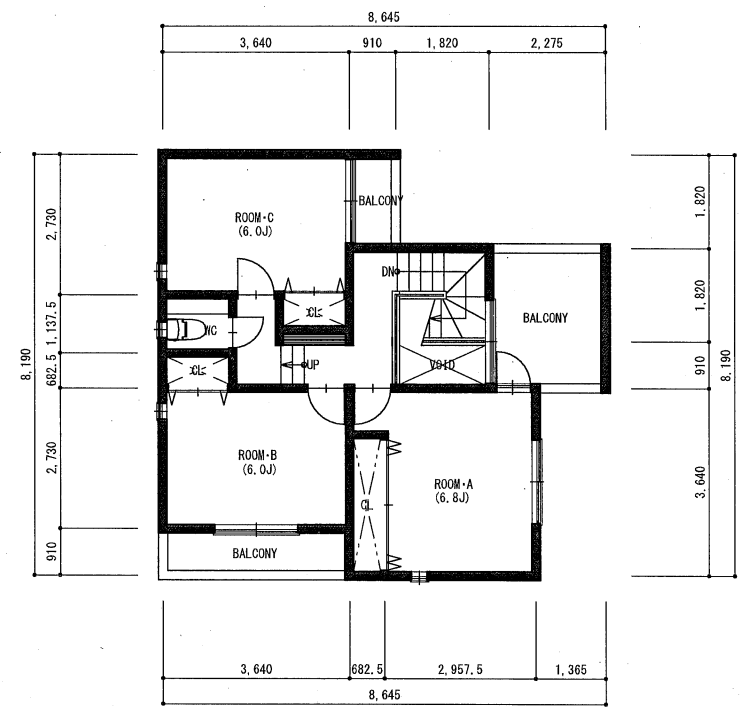
2階平面図
