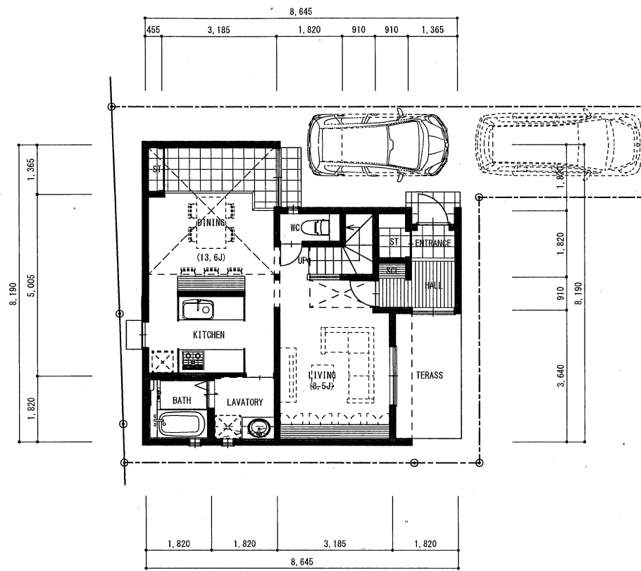
1階平面図
