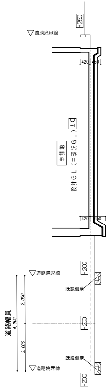
Y-Y断面図
