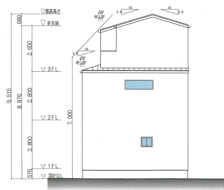
西側立面図 1/100
