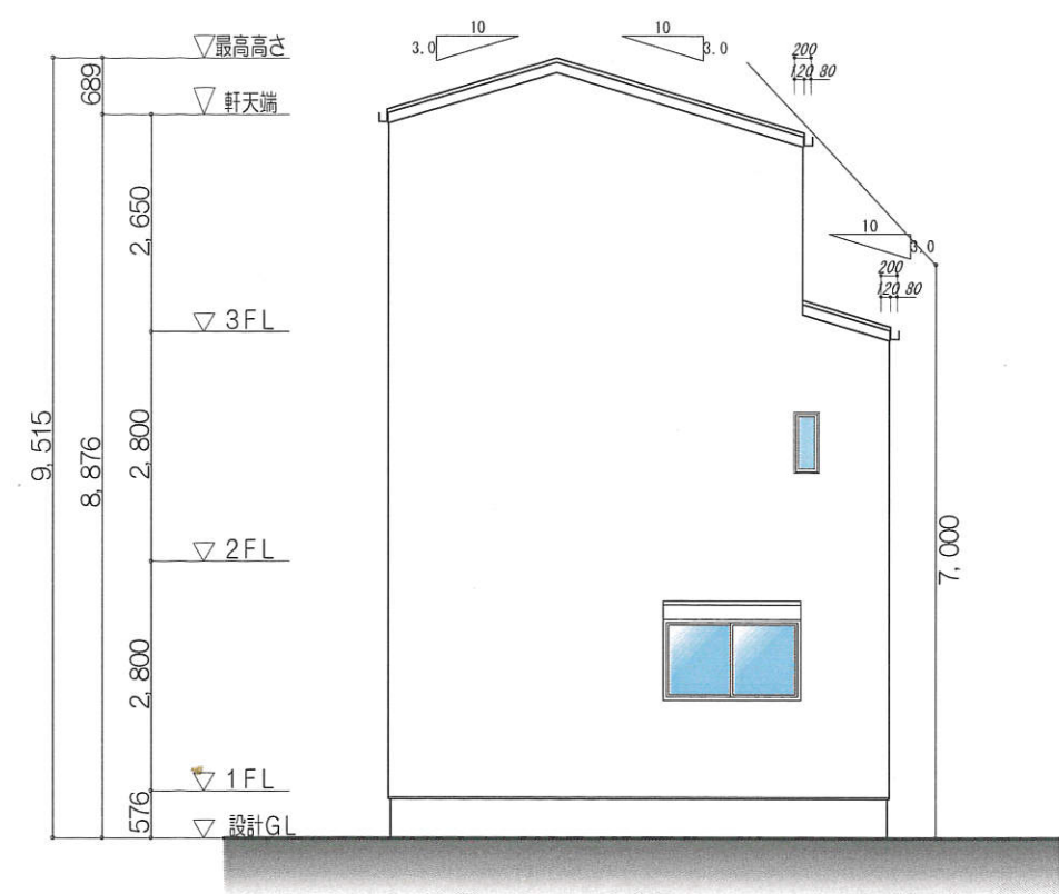
東側立面図 1/100
